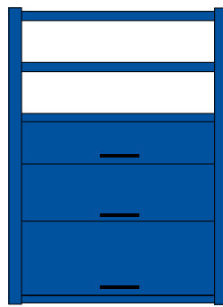
1 Fachboden 150 kg, 2 x Fachboden 500 kg, 1 x Schublade FH 250 mm, VA 500 kg, NH 120 mm, 1 x Schublade FH 350 mm, VA 500 kg, NH 220 mm, 1 x Schublade FH 450 mm, VA 500 kg, NH 320 mm, Sockelboden 50 mm
