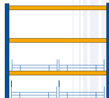
3 x Auflageholme, Tragkraft 2000 kg / Fach 2 x Palettenauszug 70 %, Tragkraft 1000 kg / Fach 2 x Palettenauszug 70 %, Tragkraft 1000 kg / Fach für Bodenmontage
