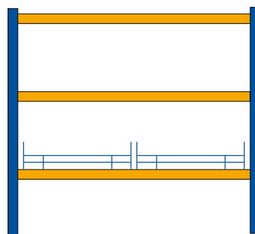
3 x Auflageholme, Tragkraft 2000 kg / Fach 2 x Palettenauszug 70 %, Tragkraft 1000 kg
